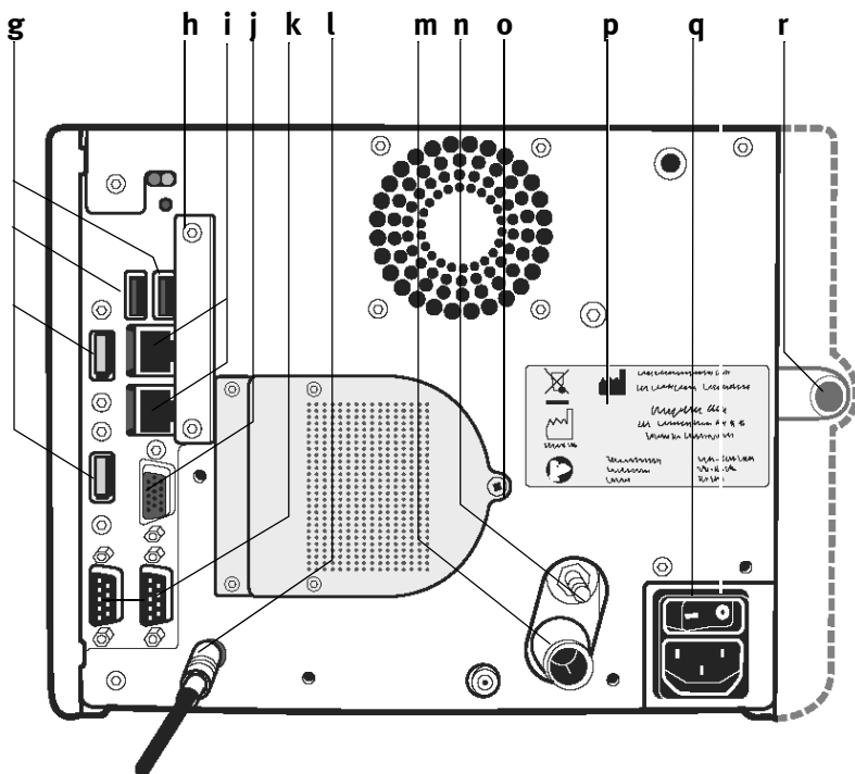
Fig. 2-2 EasyOne Pro™, rear panel
